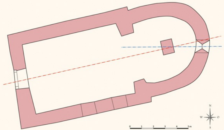
Verformungsgerechter Plan der katholischen Filialkirche Siget in der Wart.
